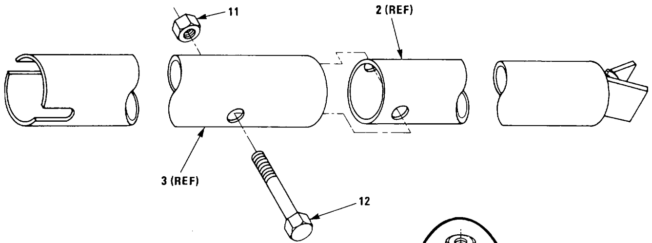
A. GIN POLE
