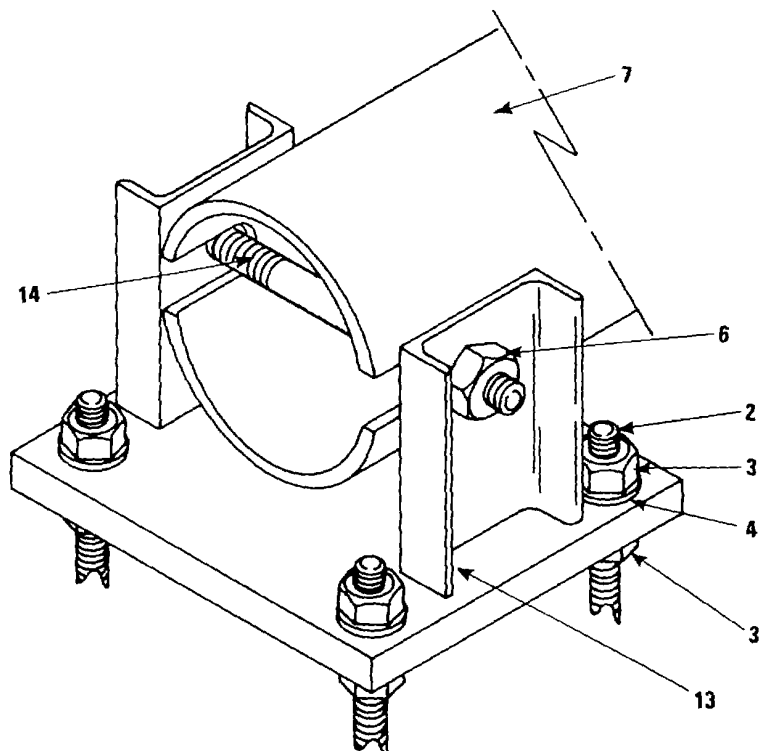
B. GIN POLE PIER
